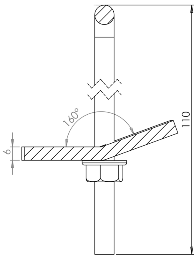
COUPE A-A
